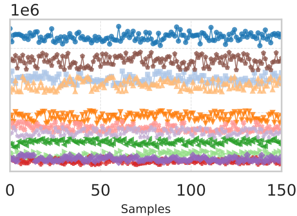
idq_uops_not_delivered.core
